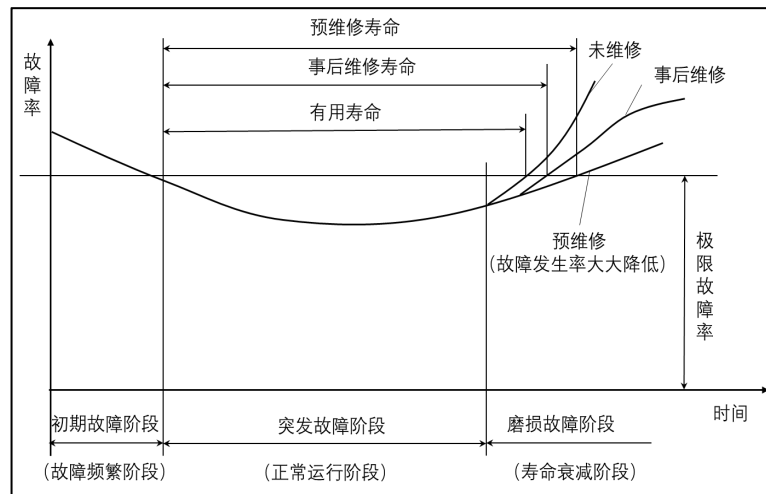
图 2 除尘设备使用寿命曲线
